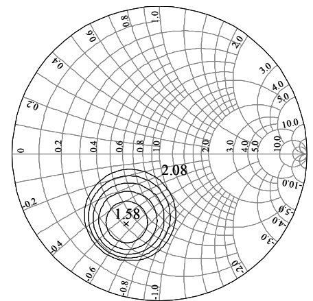
Ids=300mA
