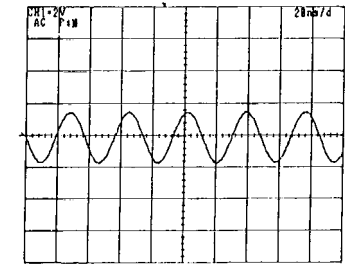
3.28 Vp-p 27 MHz
