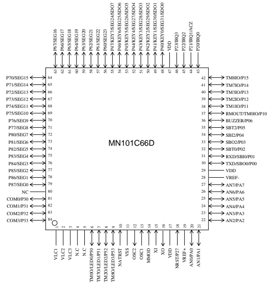
QFP084-P-1818E *Lead-free
