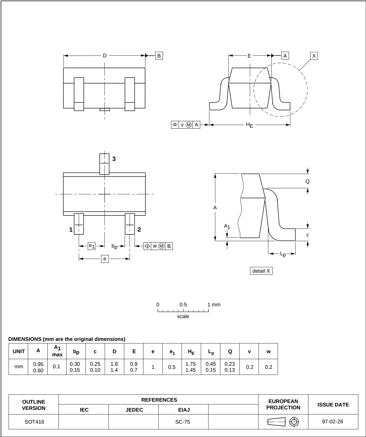
Fig 14. SOT416 (SC-75).
