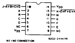
CD4002B
