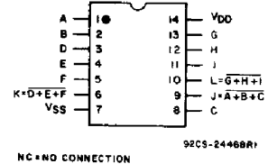
CD4025B
