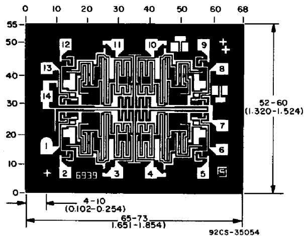
CD4001B
