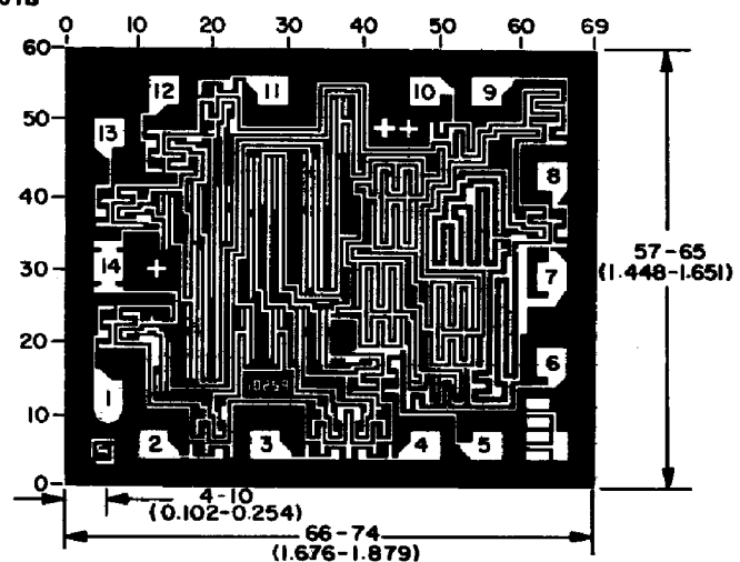
CD4025B
