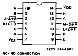
CD4001B
