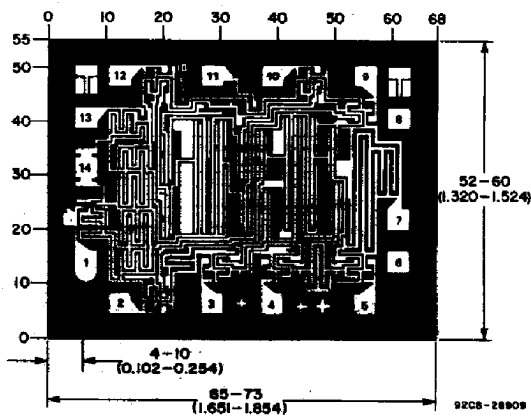
CD4002B
