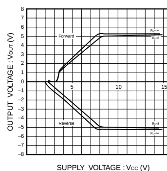
Fig.9 CH1-CH3ドライバ 電源電圧 - 出力間電圧
